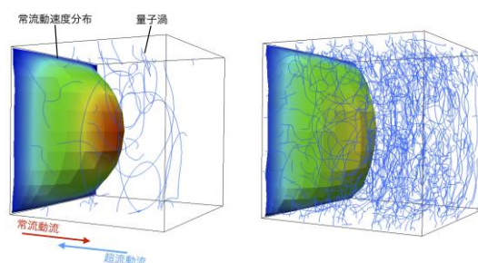
図1 量子乱流(青い線)の発達に伴い、常流動の速度分布が変形する(左図から右図へ)
